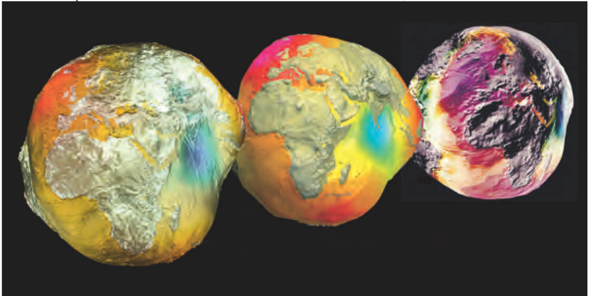
Gesteigerte räumliche Auflösung der am GFZ in den letzten Jahren berechneten Geoidmodelle: 1995 (rechts), 2005 (Mitte) und 2011 (links)
